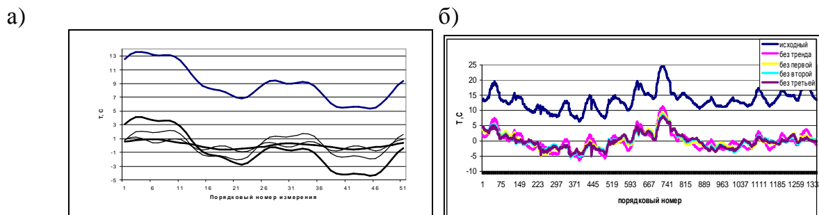
Рисунок 7. Фрагмент модельного (а) и реального (б) временного ряда – верхние кривые и временные ряды после исключения линейного тренда первой, второй и третьей периодических составляющих
