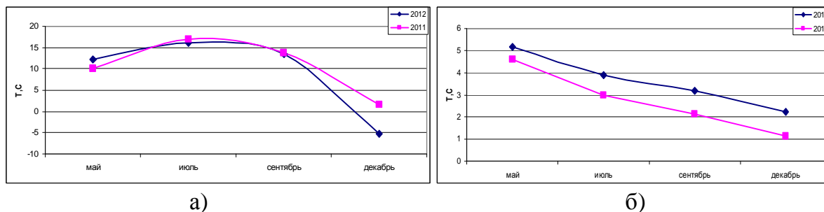
Рисунок 12. Значения средней температуры воздуха (а) и среднеквадратичного отклонения температуры воздуха от ее среднего значения (б) в Санкт-Петербурге в 2011 и 2012 гг.
