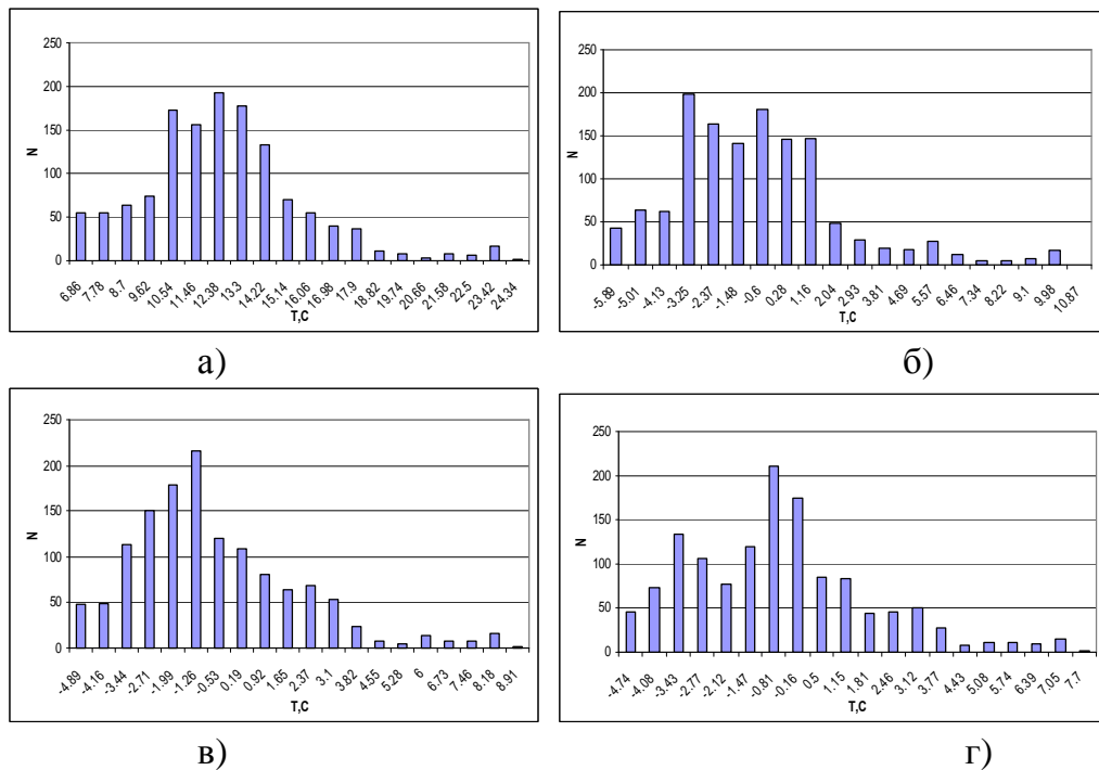
Рисунок 17. Гистограммы распределения временных рядов в процессе исключения тренда и периодических составляющих; Санкт-Петербург, 14 дней сентябрь 2012 г.
