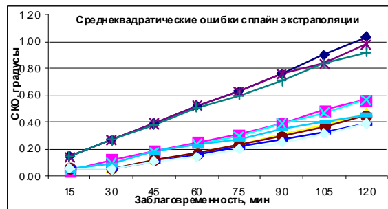
Рисунок 20. Зависимость среднеквадратических отклонений прогностических значений приземной температуры воздуха от измеренных в зависимости от заблаговременности прогнозов для сплайн экстраполяции
