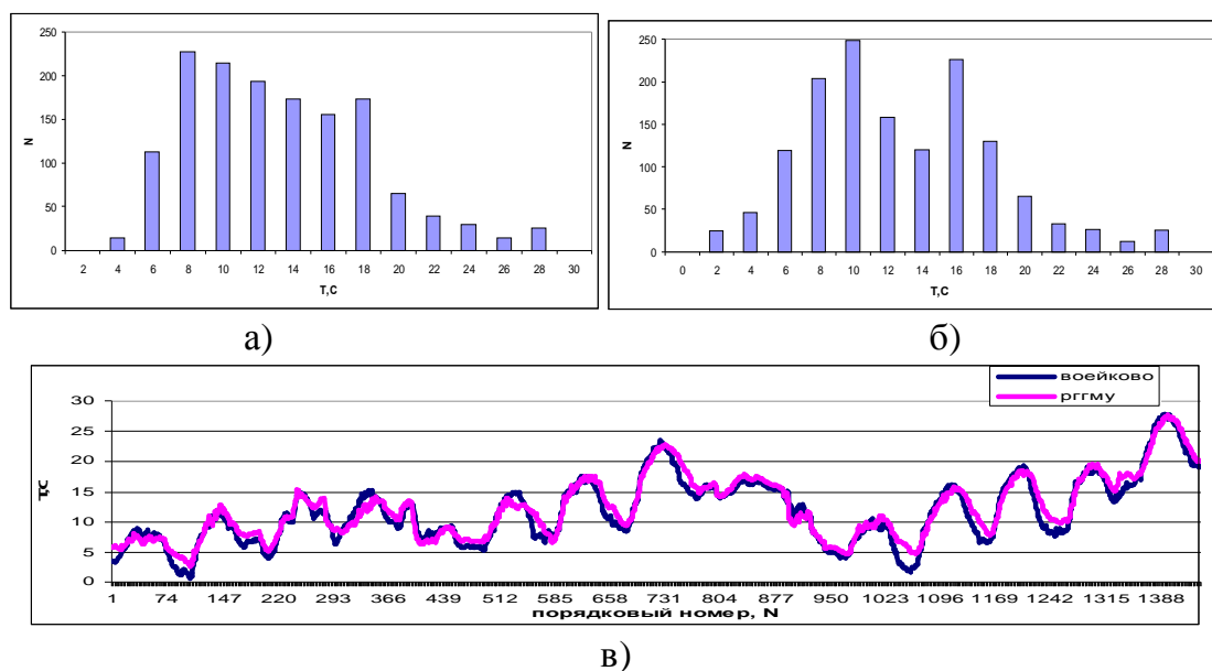
Рисунок 14. Гистограммы распределения за май 2012 г. за период 14 дней в Санкт-Петербурге (а) и Воейково (б) и ряды синхронных измерений приземной температуры воздуха в Санкт-Петербурге и Воейково (в)
