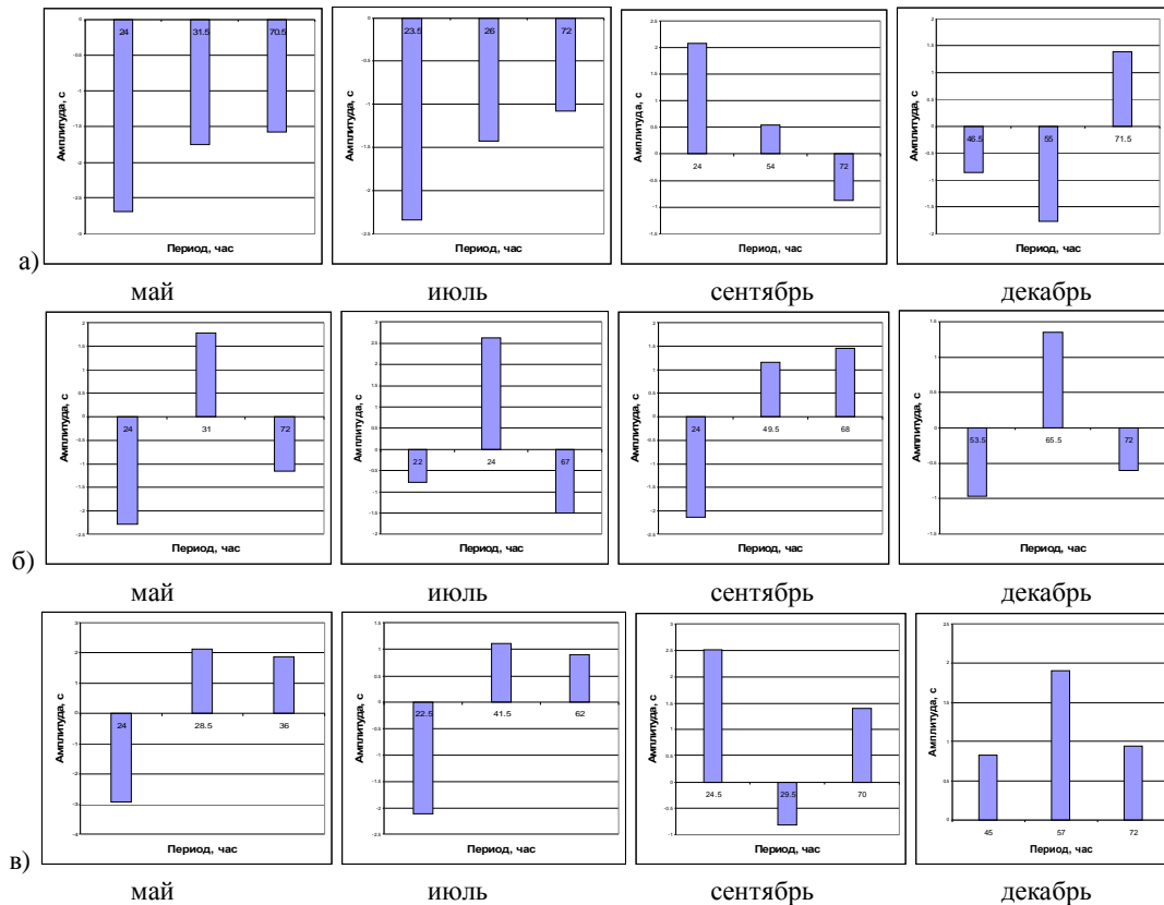
Рисунок 18. Значения амплитуды ( ^{\circ}\text{C} ) и величины периода (ч) для трех периодических составляющих для 2012 г: (а) – 14, (б) - первые 7, (в) – вторые 7 суток
