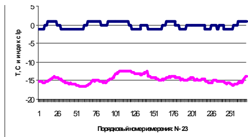
Рисунок 4. Графическое представление фрагмента временного ряда приземной температуры с дискретностью 15 мин (нижняя кривая) и функции I_p , характеризующей однородность протекаемого процесса (верхняя кривая)
