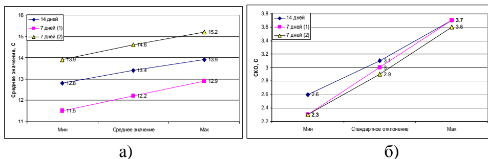
Рисунок 13. Средние значения (а) и среднеквадратичные отклонения (б) температуры с 95% доверительными интервалами в Санкт-Петербурге за сентябрь 2012 г, вычисленные по фрагментам временного ряда, содержащим 14, 7 (1), и 7 суток (2)
