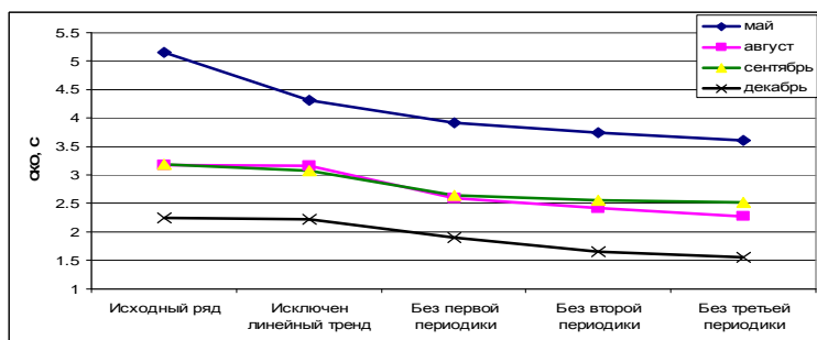
Рисунок 16. Изменение величины среднеквадратичного отклонения в процессе исключения линейного тренда и трех периодических составляющих для мая, августа, сентября и декабря 2012 г (14 суток)
