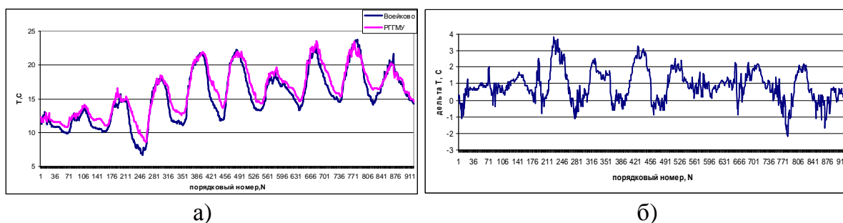
Рисунок 11. Фрагмент временных рядов приземной температуры воздуха за август 2012 г, измеренной АМС в Санкт-Петербурге РГГМУ и Ленинградской области, Воейково ИРАМ (а), и разность температур ( \Delta T ) между ними (б)
