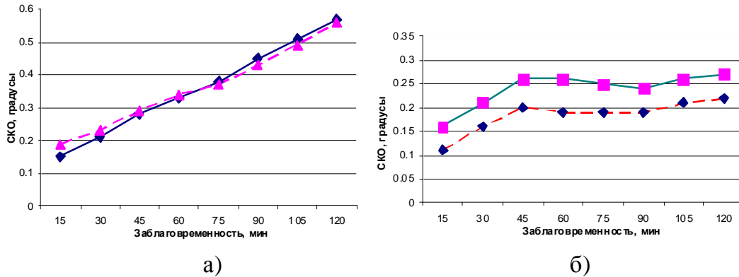
Рисунок 19. Зависимость среднеквадратических отклонений прогностических значений приземной температуры воздуха от измеренных по данным АМС.
