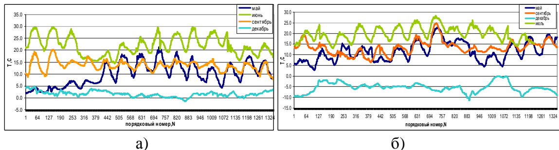
Рисунок 8. Временные ряды приземной температуры воздуха, измеренной АМС РГГМУ, за 4 месяца 2011 г. (а) и 2012 г. (б)
