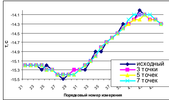
Рисунок 5. Исходный временной ряд приземной температуры и сглаженные по 3, 5 и 7 точкам ряды
