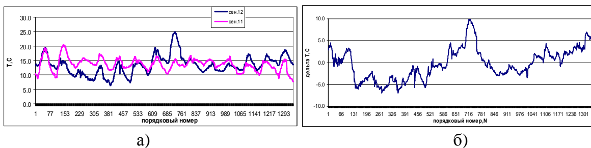
Рисунок 9. Сопоставление временных рядов приземной температуры воздуха за сентябрь месяц 2011 и 2012 гг. (а) и значений \Delta T ; (б) за тот же период
