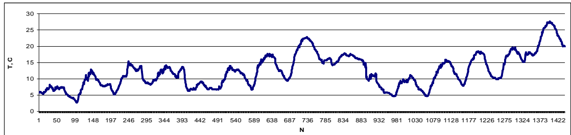
Рисунок 1. Фрагмент временного ряда приземной температуры воздуха за май 2012 года
