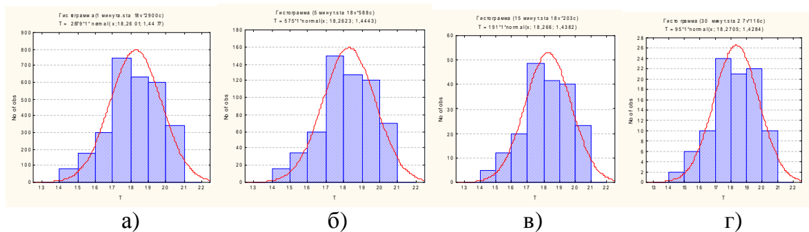
Рисунок 3. Гистограммы распределения значений температуры воздуха за 30–31 июля 2011 г. при различной дискретности измерений: а) 1 мин; б) 5 мин; в) 15 мин; с) 30 мин
