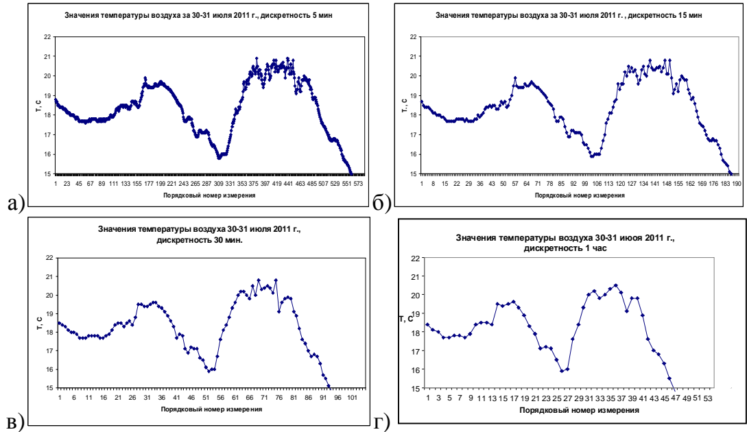
Рисунок 2. Графическое представление временного ряда приземной температуры с различной дискретностью: а) 5 мин, б) 15 мин, в) 30 мин, г) 60 мин
