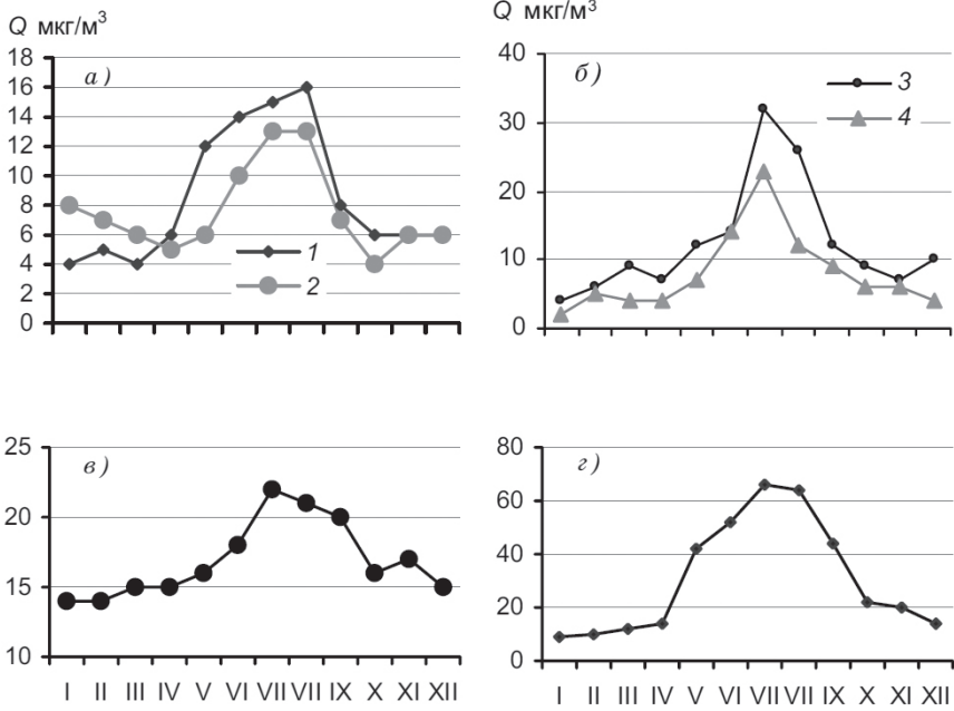
Рис. 1. Годовой ход концентрации формальдегида в городах. а — Казань (1) и Тольятти (2), б — Дзержинск (3) и Сыктывкар (4), в — Ставрополь, з — Ясная Поляна.
