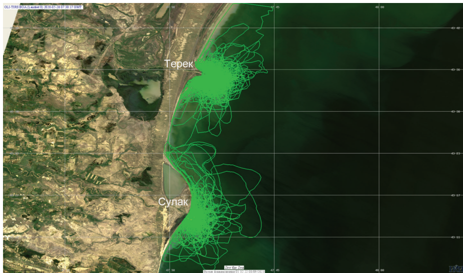
Рисунок 11 — Сводная карта границ плуомов рек Терек и Сулак, выявленных по спутниковым данным видимого диапазона за 2014–2022 гг.
