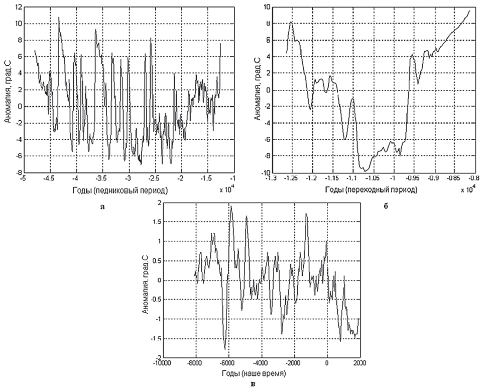
Рис. 3. Ряды аномалий температуры в центральной части Гренландии по трем временным периодам с дискретностью 30 лет.
