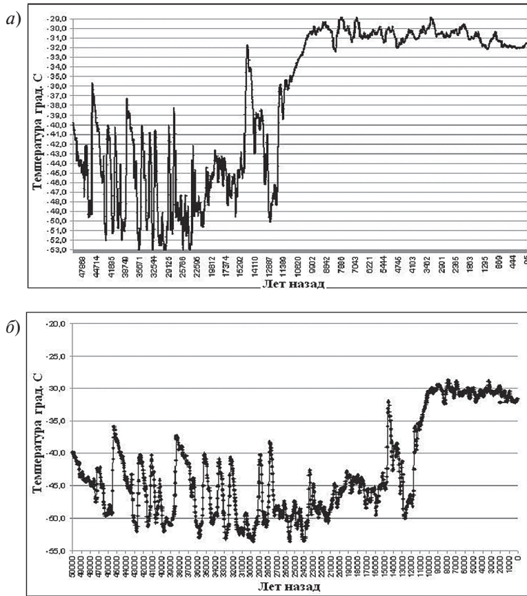
Рис. 1. Реконструированные данные температуры в центральной части Гренландии за последние 50 000 лет (а) и преобразованный ряд реконструированных данных температуры (б) с дискретностью 30 лет (длина ряда составляет 1661 значение).
