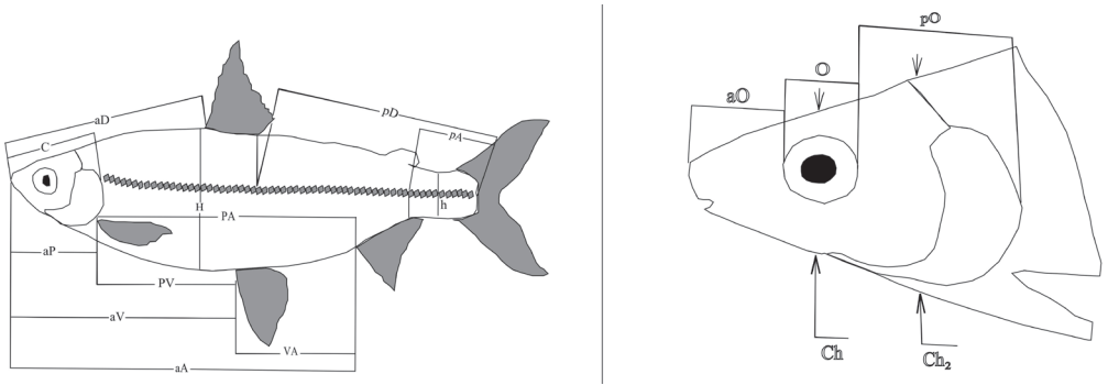
Рис. 2. Схема промеров рыб отряда лососеобразных по Смитту, с изменениями [20].
